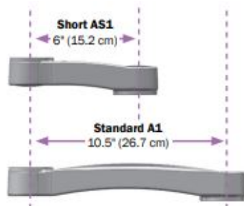
水平アーム
