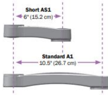
延長アーム
